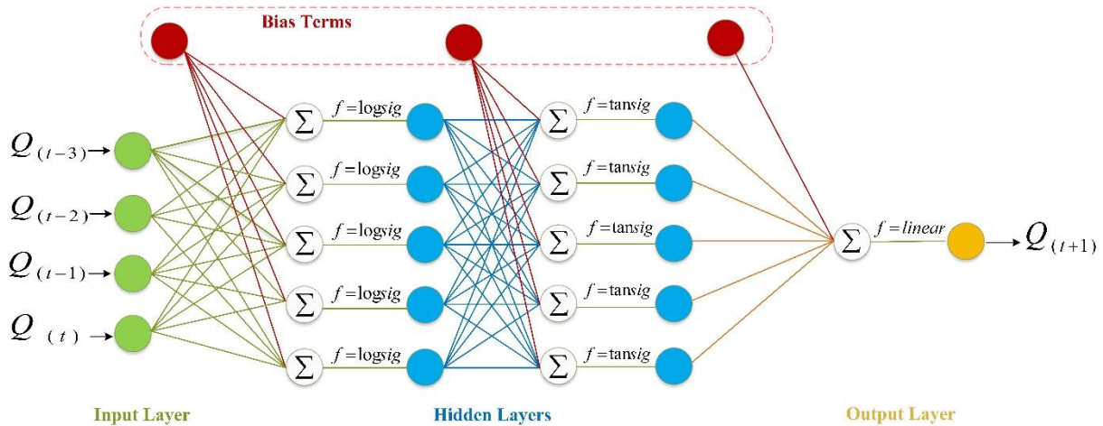
شکل ۴- شبکه عصبی مصنوعی سه لایه با معماری ۱-۵-۵-۴
